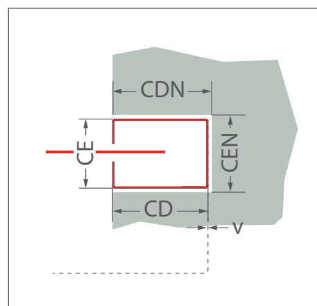
Nischenmontage
