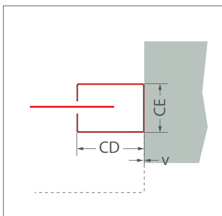
Laibungsmontage
